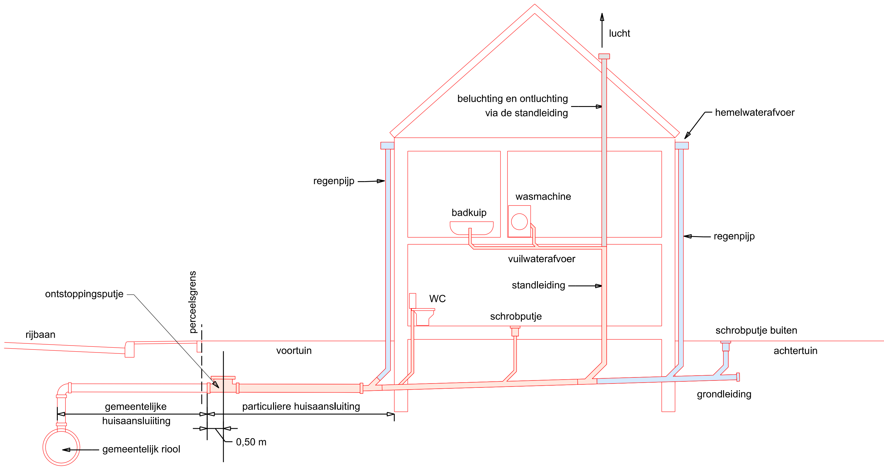
Principeschets rioolaansluitleiding woning
