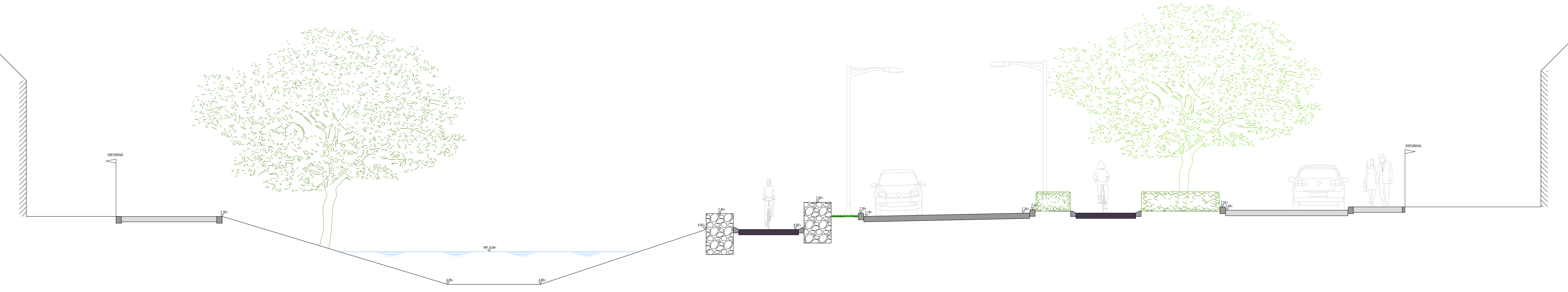
DOORSNEDE A-A SCHAAI 1:50
