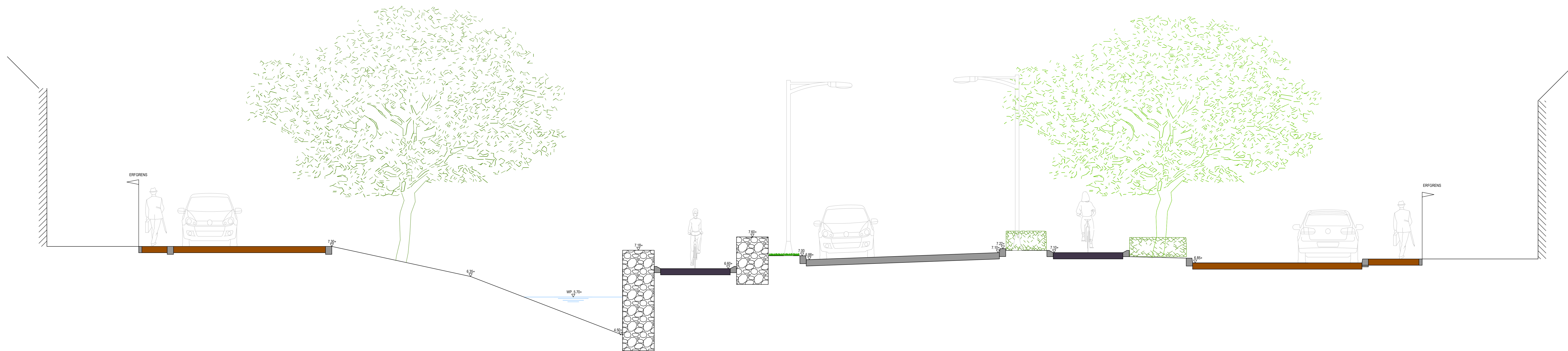
DOORSNEDE C-C SCHAAI 1:50
