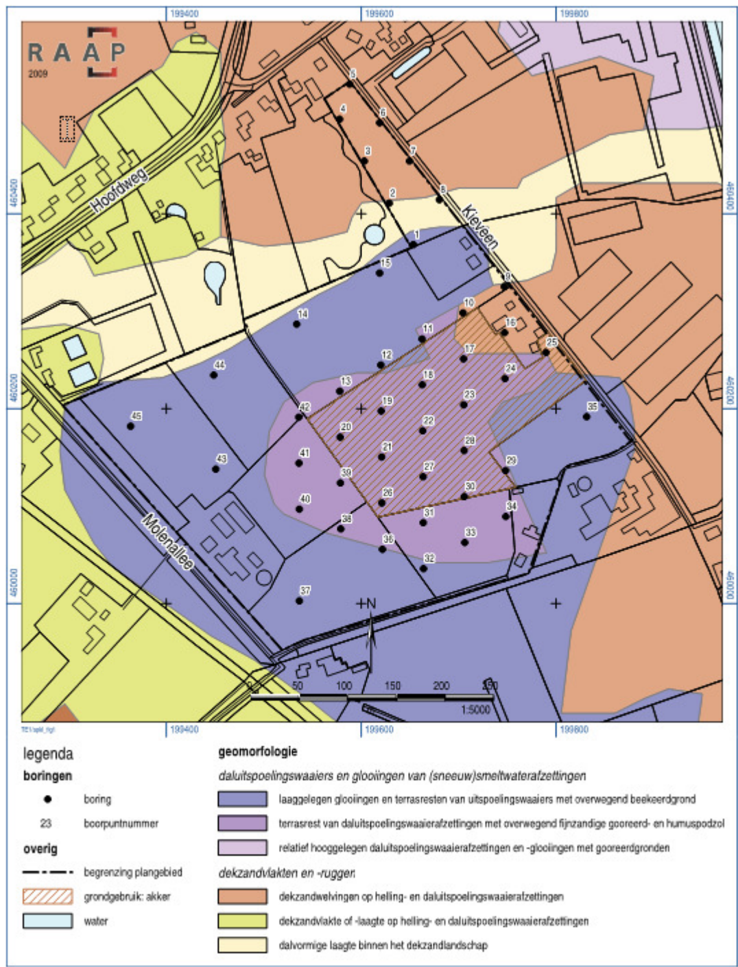
Figuur 1. Boorpuntenkaart, weergegeven op de geomorfologische kaart van Apeldoorn (bron: RAAP-rapport 1131).
